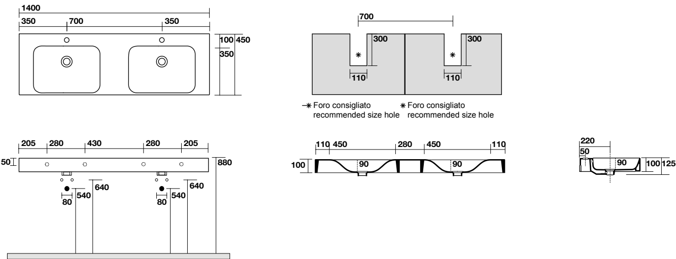
3536 Lavabo 140x45 cm doppia vasca sospeso, appoggio monoforo. 140x45 cm single hole, wall-hung or countertop double basin.
