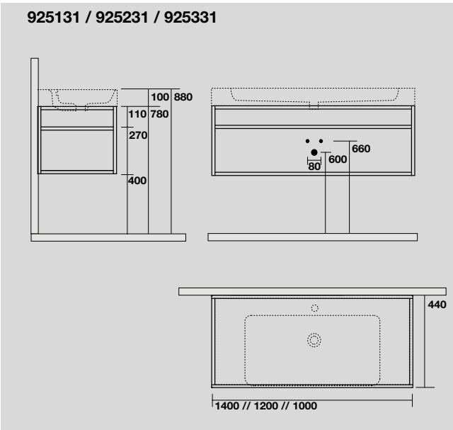
925331 Struttura sospesa in acciaio con ripiano in metallo nero matt per lavabo cm 140x45 cm con ripiani laterali. Wall-hung matt black steel vanity unit with metal shelf prepared for 140x45 cm washbasin with side shelf space.
