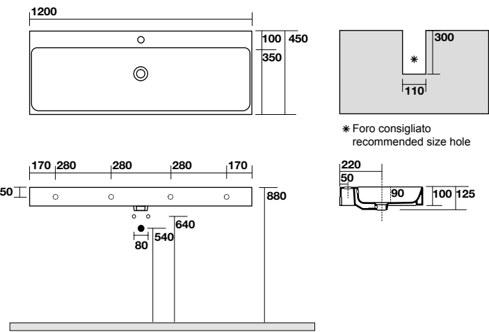
3534 Lavabo monoforo 120x45 cm sospeso o appoggio. 120x45 cm single hole wall-hung or countertop basin.
