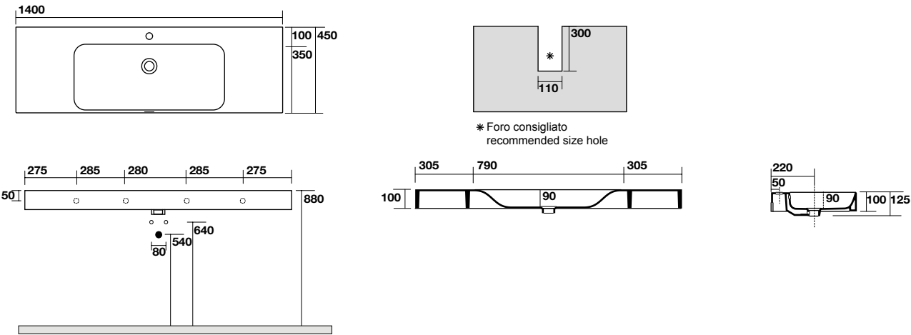
3535 Lavabo 140x45 cm con piani laterali, sospeso o appoggio monoforo. 140x45 cm single hole wall-hung or countertop basin with side shelf space.
