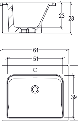
Vasca L. 51 x 39 cm per top P. 62,5 / 68,5 cm
