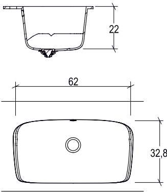
Vasca L. 62 x 32,8 cm per top P. 50,5 cm
