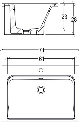
Vasca L. 61 x 39 cm P. 62,5 / 68,5 cm
