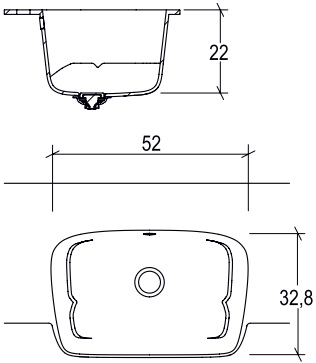
Vasca L. 52 x 32,8 cm per top P. 36,5 cm
