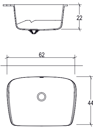
Vasca L. 62 x 44 cm per top P. 62,5 / 68,5 cm
