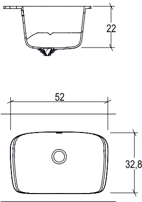
Vasca L. 52 x 32,8 cm per top P. 50,5 cm
